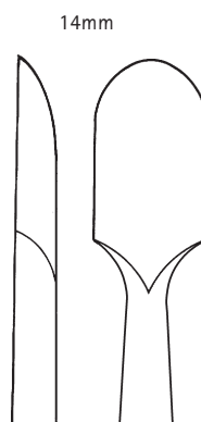
FK324R 骨膜剥離子 直 幅 14mm 195mm vb00145
